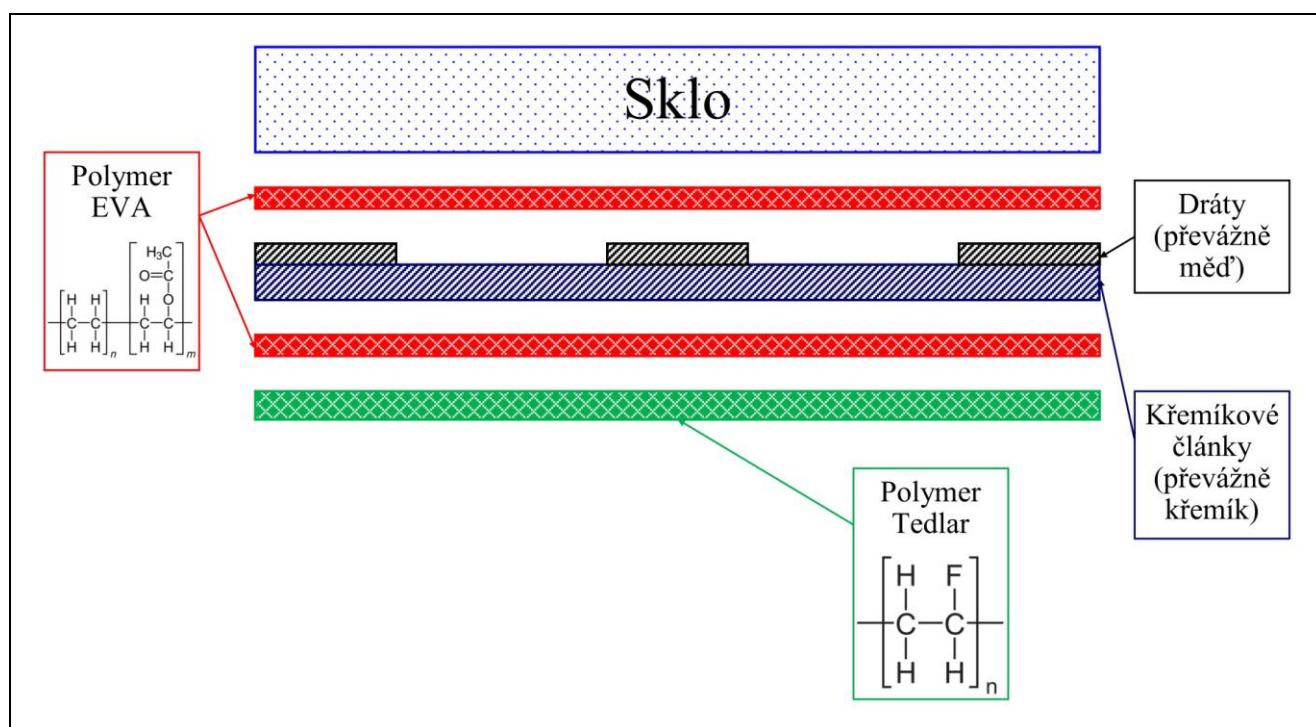
Obr. 1: Typická struktura solárního fotovoltaického panelu křemíkového typu.
